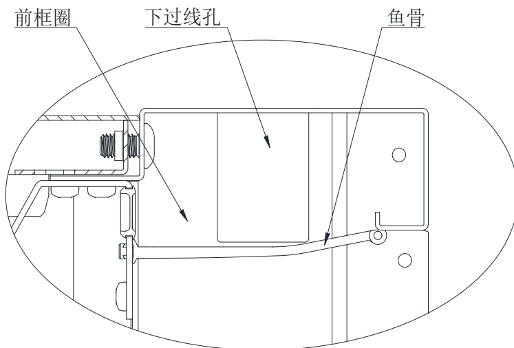
图 21: 600 宽机柜前部走线槽示意图
