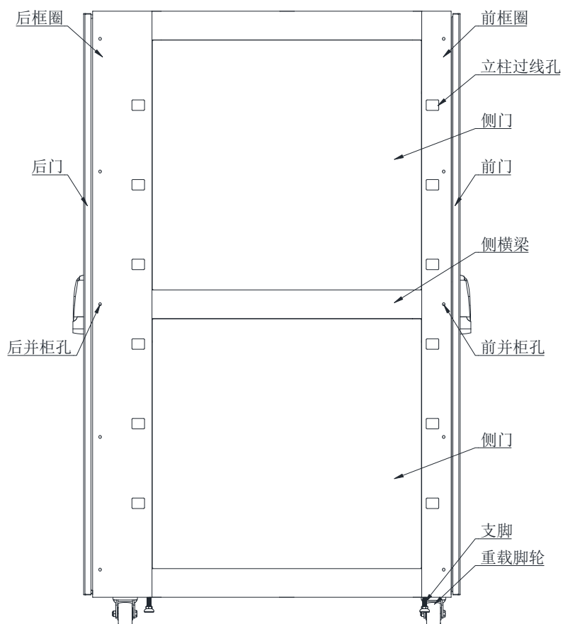
图 26: 机柜侧面示意图
