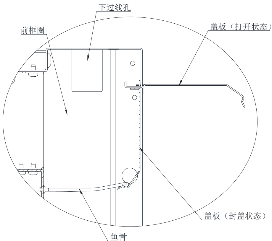
图 22: 800 宽机柜前部走线槽示意图
