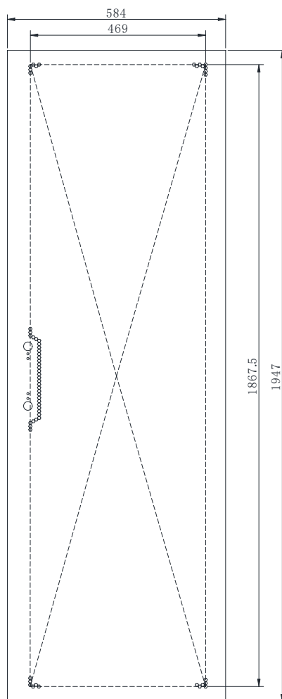
图 12: 机柜门板开孔区域示意图
