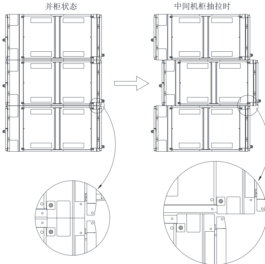
图 36: 并柜机柜抽拉示意图
