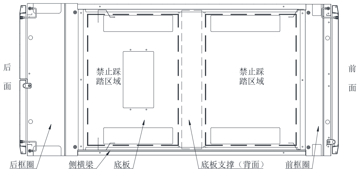
图 9: 机柜底部禁止踩踏区域示意图
