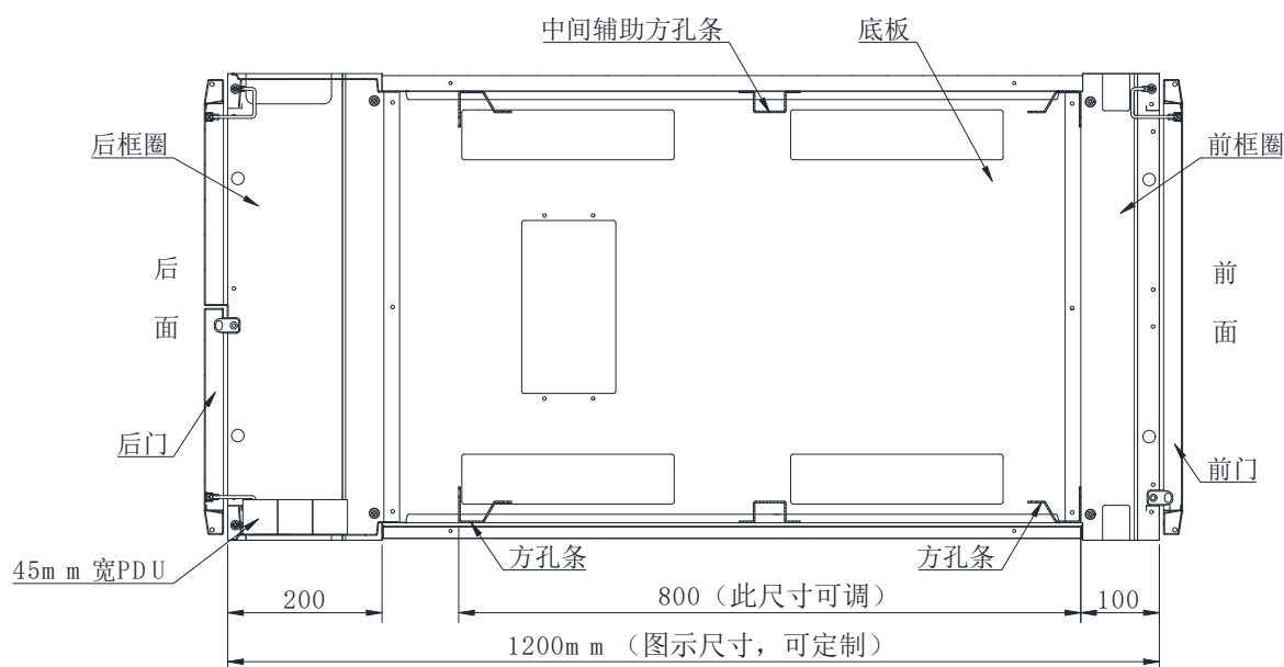
图 17: 机柜内部方孔条安装位置示意图
