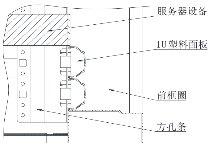
图 13: 机柜前腔密封示意图
