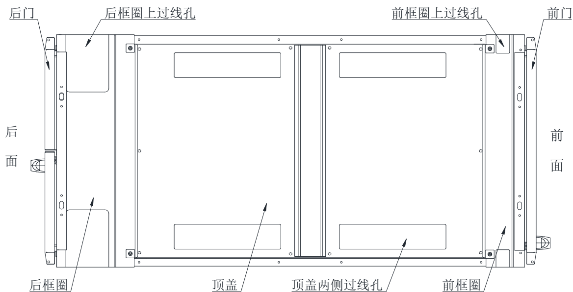
图 24: 机柜顶部过线孔位置示意图
