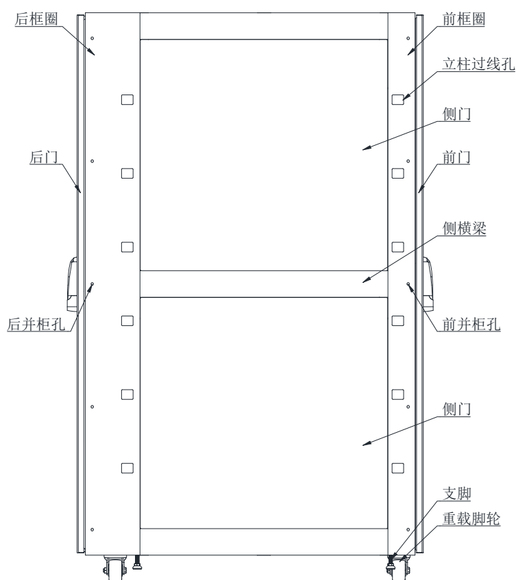
图 38：机柜两段式侧门示意图
