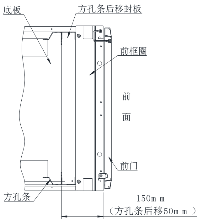
图 14: 机柜方孔条后移密封示意图
