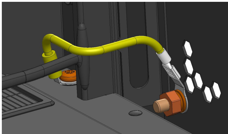
图 10：机柜内部接地线组件连接示意图
