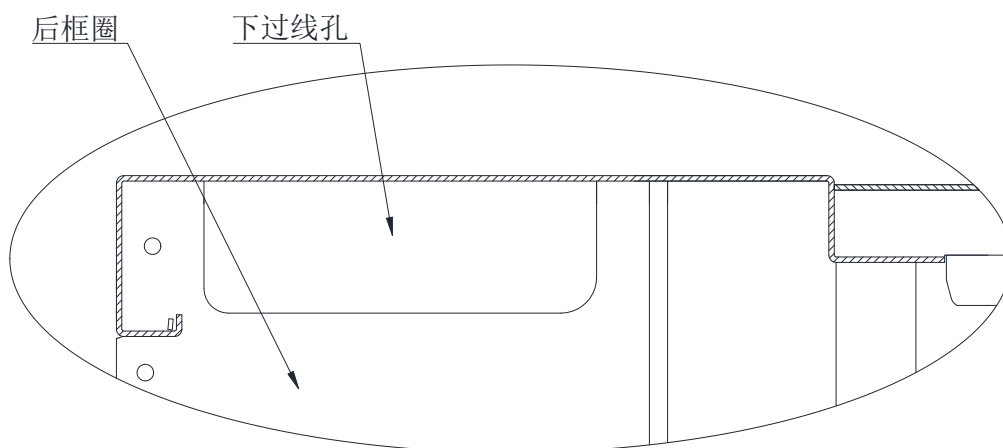
图 23: 机柜后部走线槽示意图
