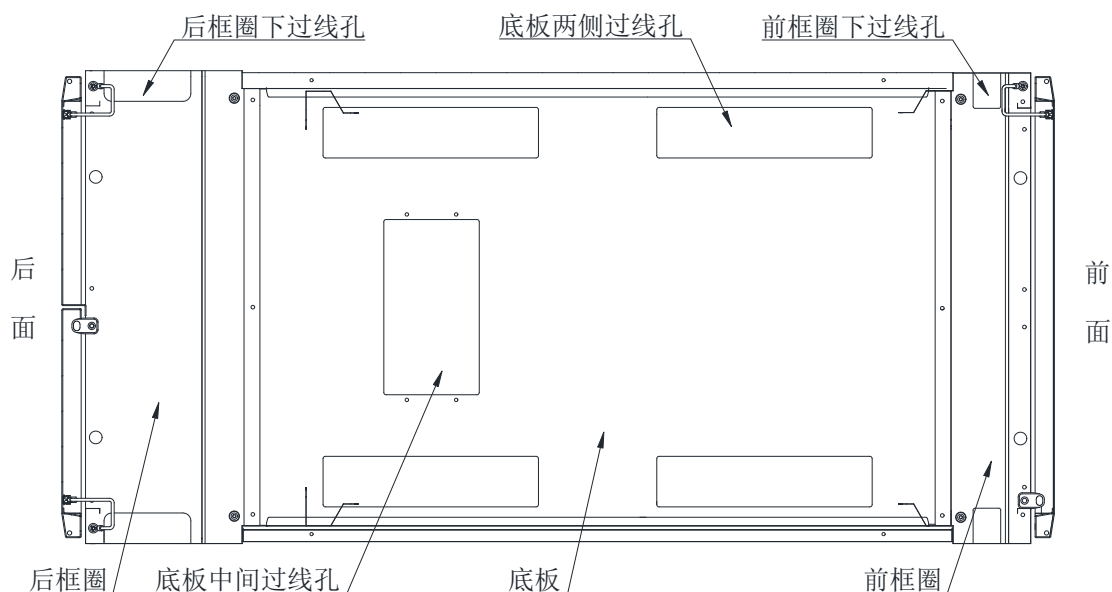
图 25: 机柜底部过线孔位置示意图
