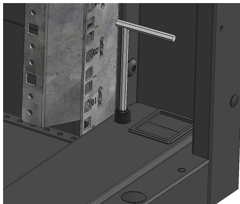
图 37: 机柜内部调节支脚高度示意图
