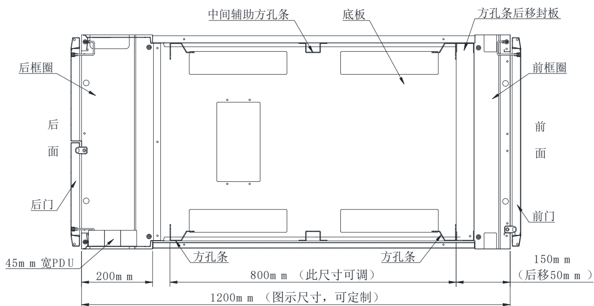
图 18: 机柜内部方孔条移位安装位置示意图
