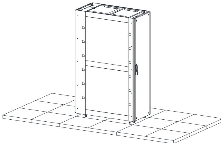
图 34：机柜带脚轮/支脚安装于静电地板上示意图
