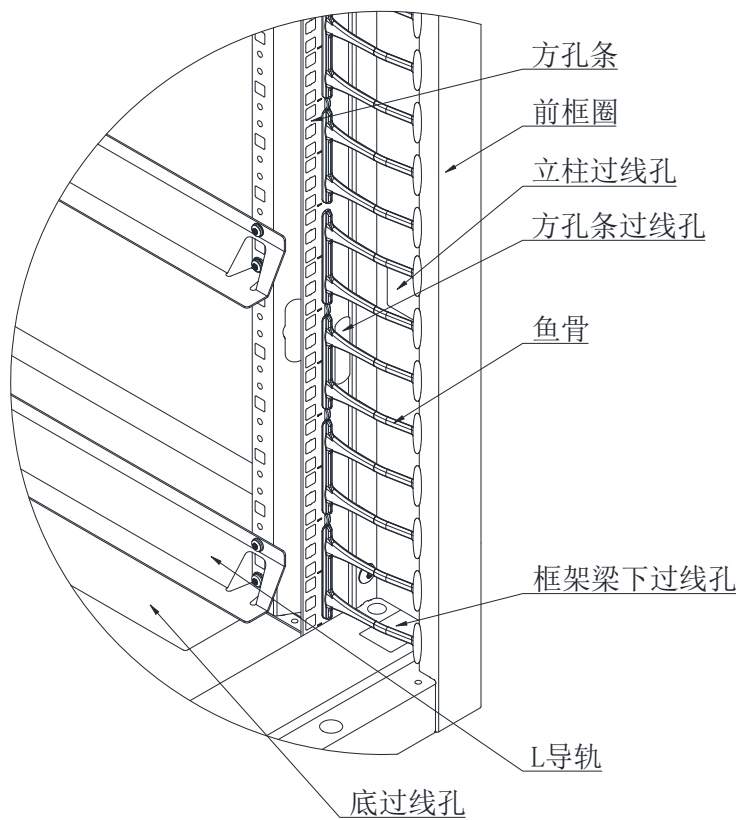
图 27: 机柜内部过线孔位置示意图
